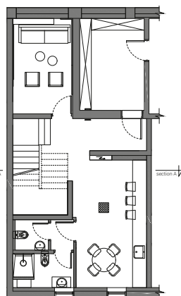
Grundriss Untergeschoss • Basement floor plan
